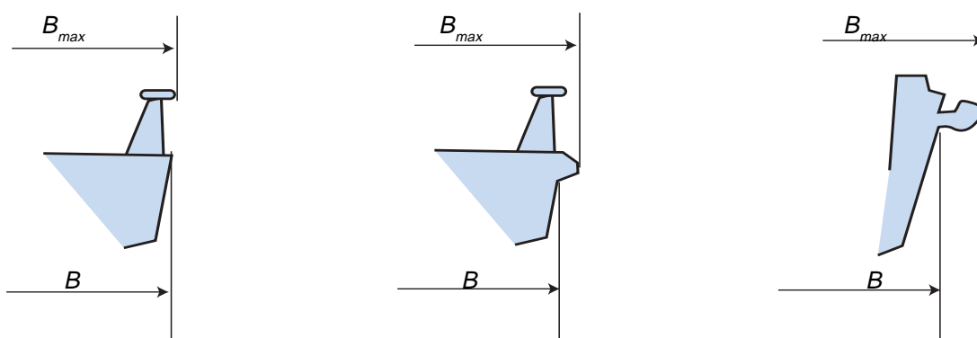
Figur 9.4. Mätning av maximal bredd B_{max} .
