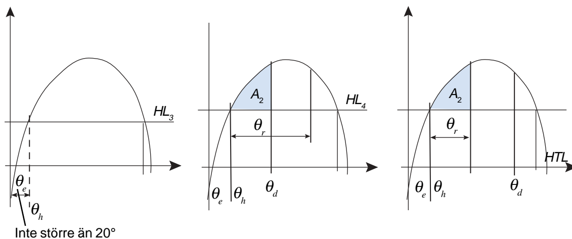
Figur 2. Läckstabilitet.
