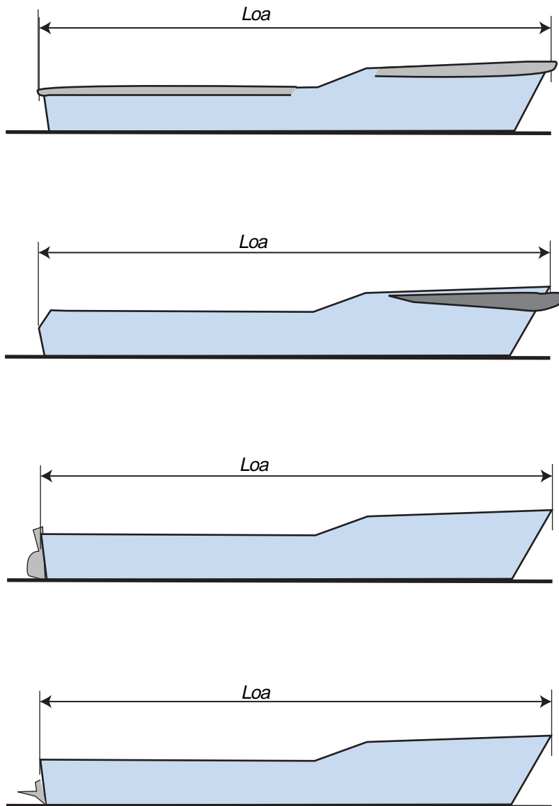
Figur 9.3. Mätning av längd över allt L_{oa} .
